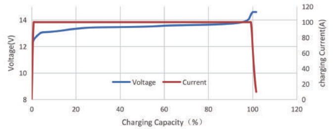
LADEZUSTANDSKURVE (0,5C, 25°C)
