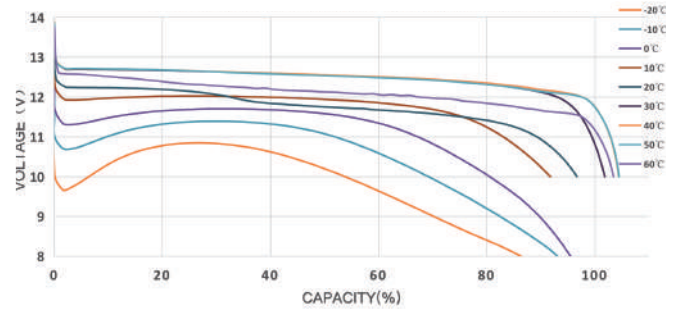
UNTERSCHIEDLICHE TEMPERATURENTLADUNGSKURVE (0,5C)
