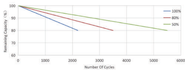
UNTERSCHIEDLICHE DOD-ENTLADUNGSZYKLUS-LEBENS-KURVE (0,5 C)
