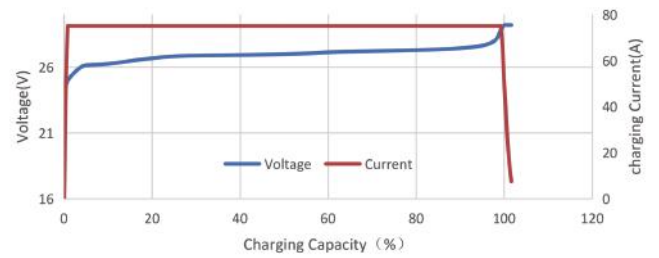
LADEZUSTANDSKURVE (0,5C, 25°C)
